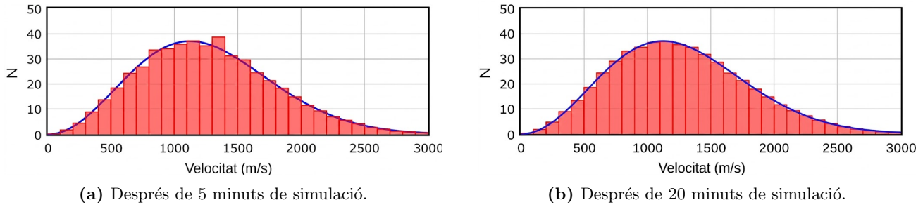
Figura 1.7: Distribució de velocitats per r_0 = 0,04 m.
