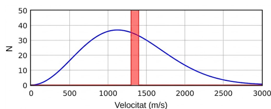
Figura 1.2: Distribució de velocitats per r_0 = r_{real} després de 5 minuts de simulació.
