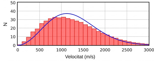
Figura 1.4: Distribució de velocitats per r_0 = 0,1 m després de 5 minuts de simulació.
