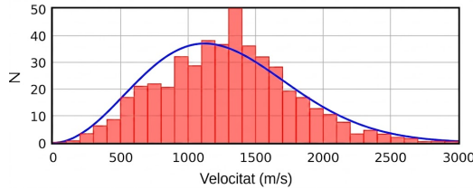
Figura 1.5: Distribució de velocitats per r_0 = 0,01 m després de 5 minuts de simulació.
